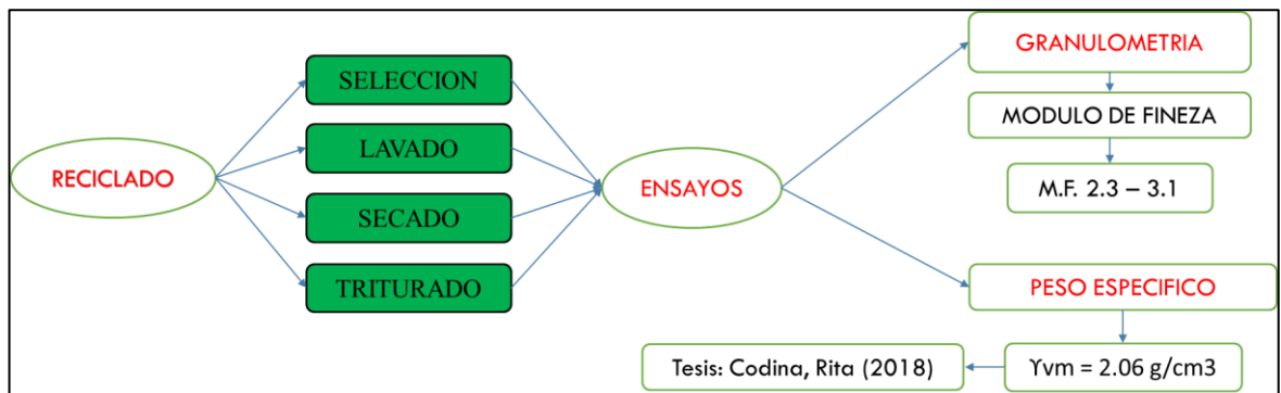
Figura 3. Pasos para la caracterización del vidrio reciclado
