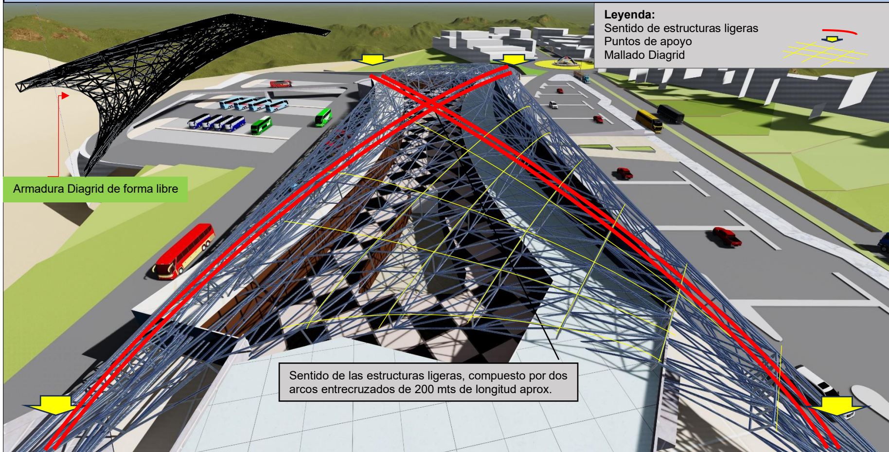
Figura 80. Diseño estructural de cobertura Diagrid de forma libre.
