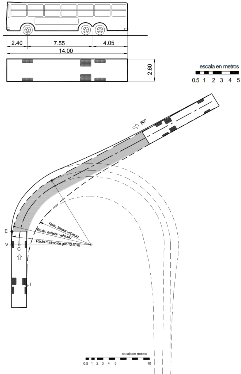
Figura 48. Radios de giro de un Ómnibus de tres ejes (B2); (Fuente: Manual de carreteras Diseño Geométrico DG - 2018).
