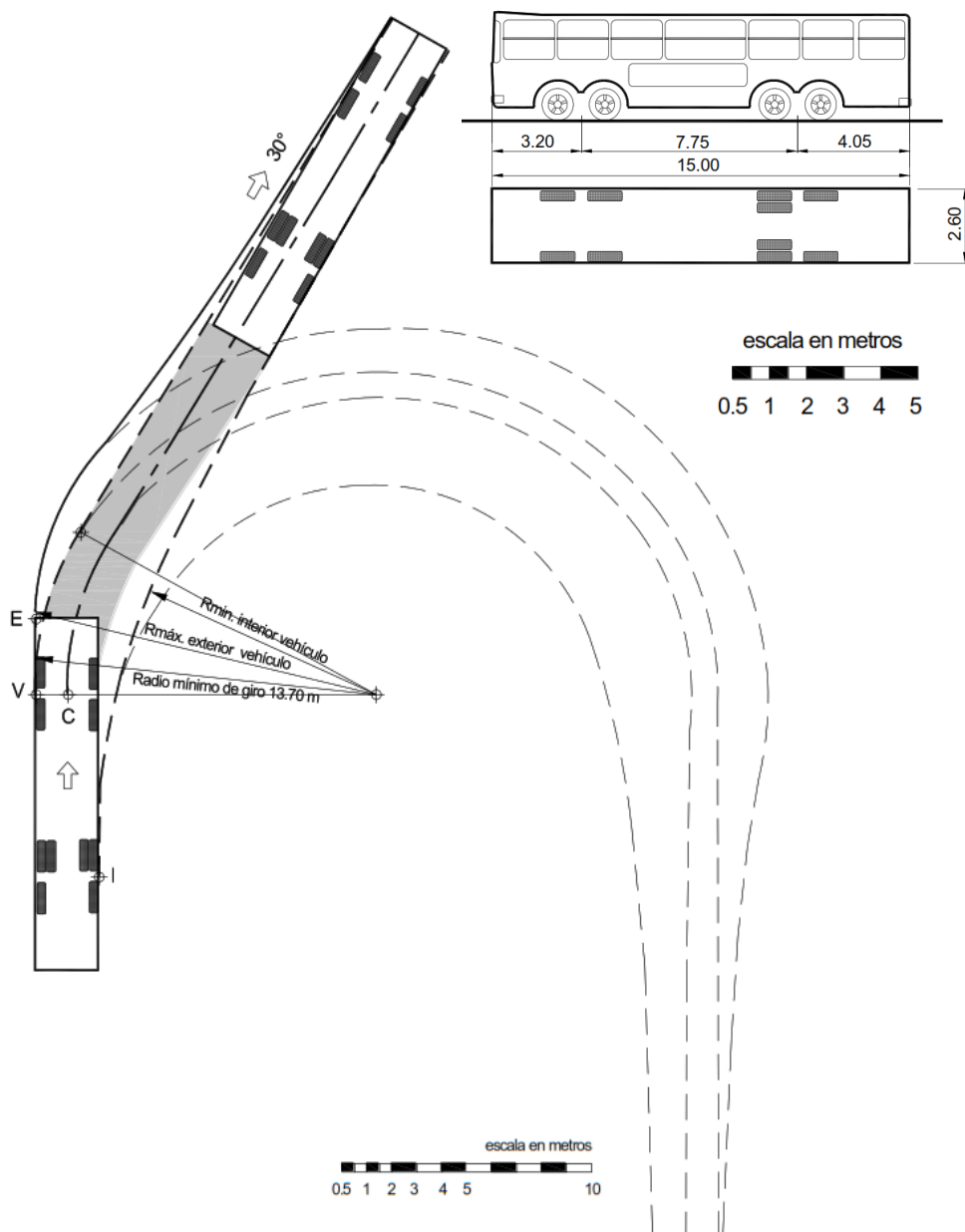
Figura 49. Radios de giro de un Ómnibus de cuatro ejes (B2); (Fuente: Manual de carreteras Diseño Geométrico DG - 2018).
