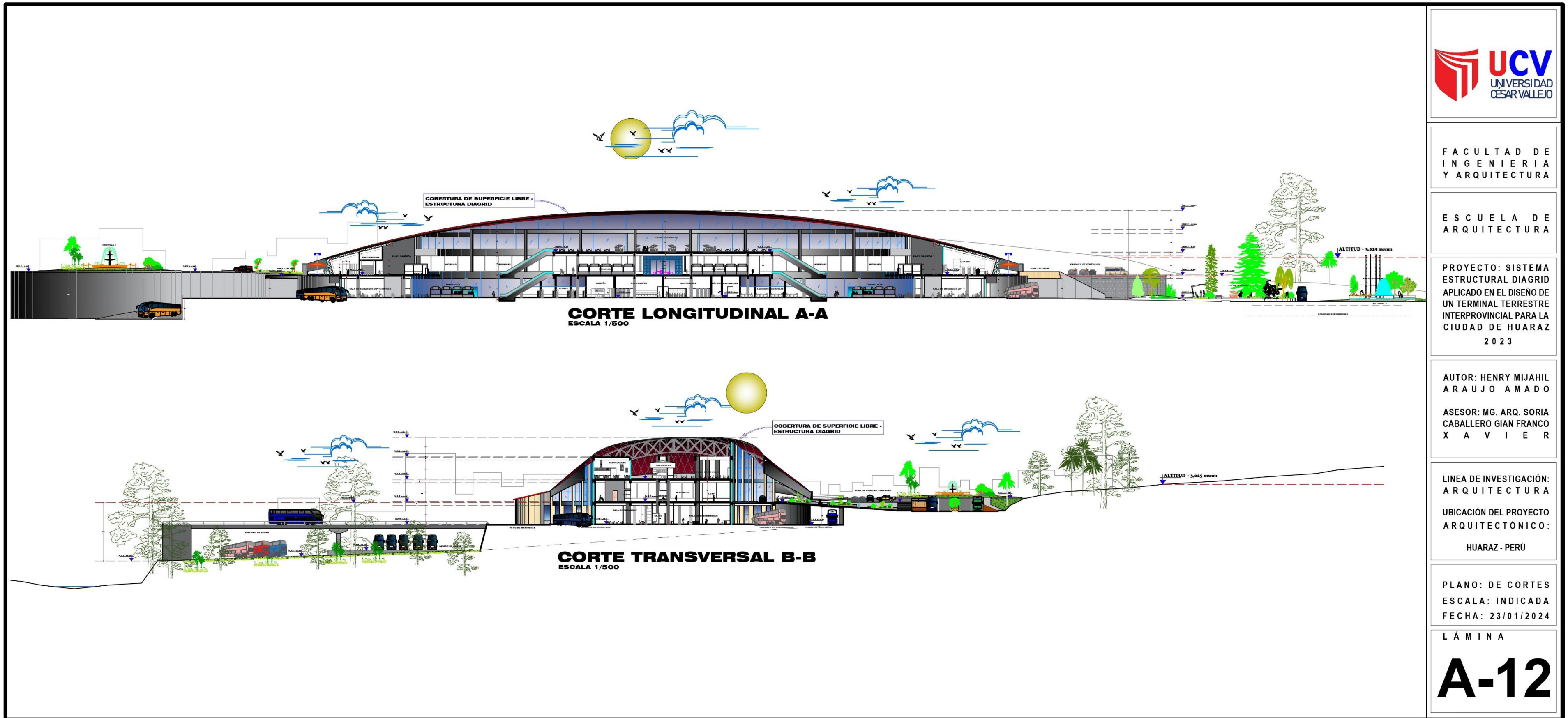
Figura 106. Plano de cortes
