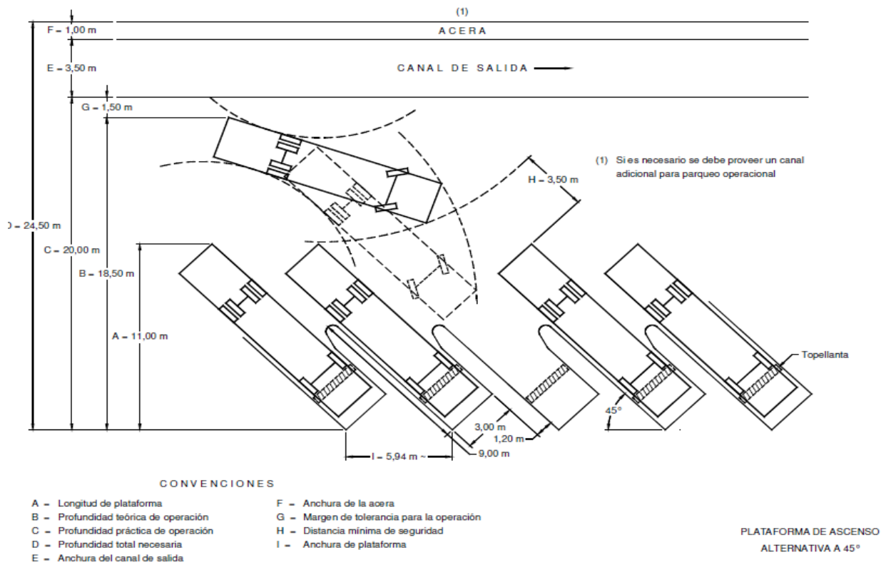
Figura 41. Tipología de medidas y giros en andenes con una inclinación de 45°; (Fuente: Regconomica_Proyecto Norma Técnica Colombiana 430 04).
