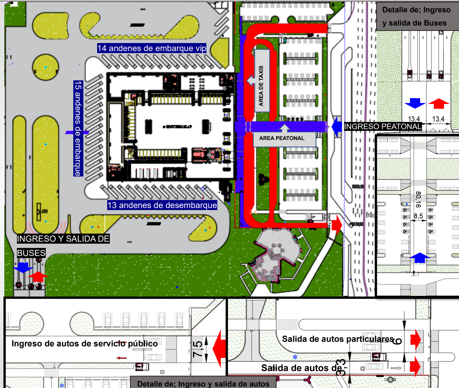
Figura 70. Terminal terrestre de Trujillo, análisis arquitectónico funcional
