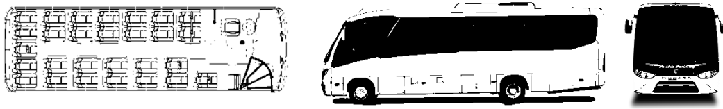
Figura 50. Minibús de 29 pasajeros de dos ejes; (Fuente: Catálogo Marcopolo)
