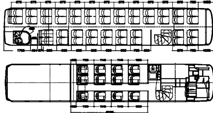
Figura 53. Autobús de 60 pasajeros de tres ejes; (Fuente: Catálogo Marcopolo)
