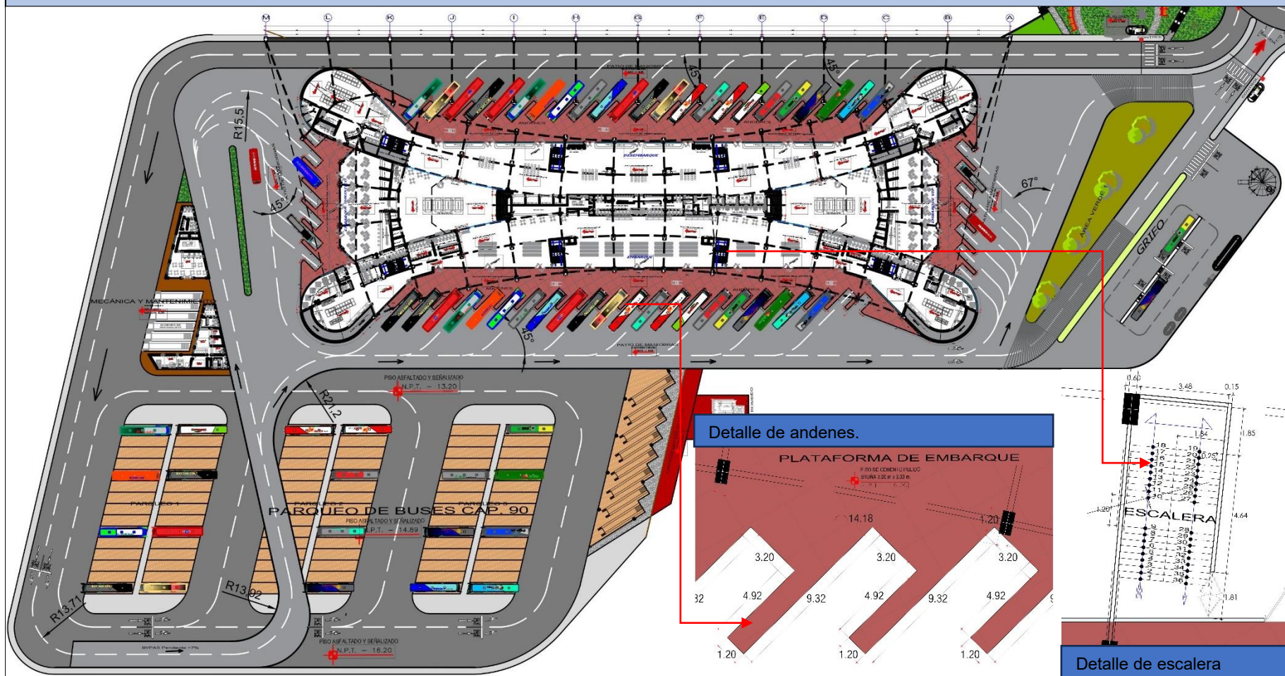
Figura 85. Proceso de diseño; primer nivel.
