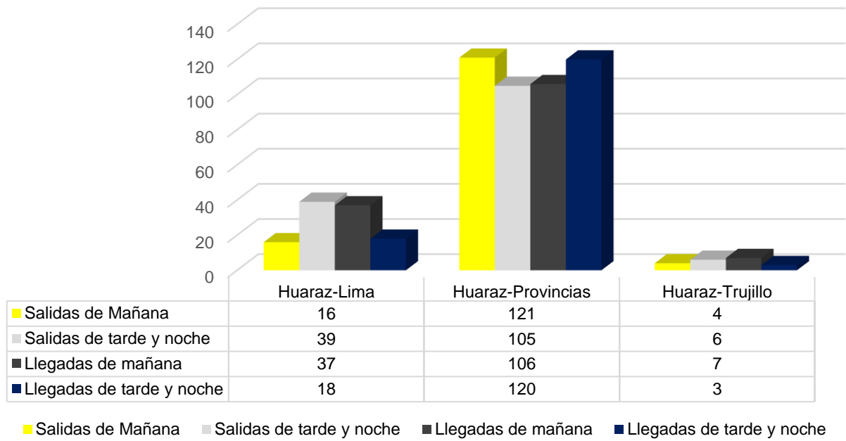
Figura 7. Análisis general; de salidas y llegadas diarias de las empresas del transporte interprovincial en Huaraz.
