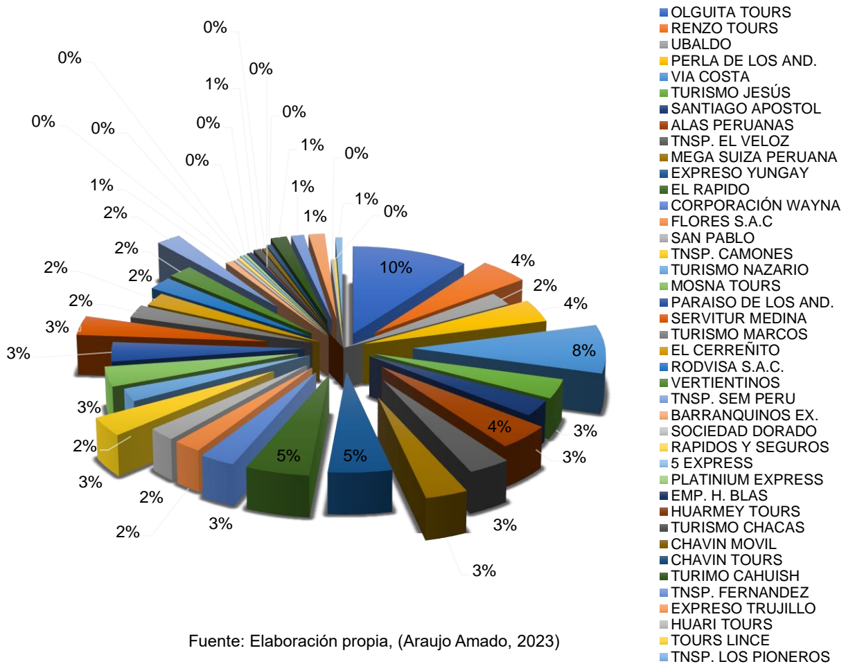
Figura 9. Porcentaje del movimiento de pasajeros por empresa; de acuerdo a salidas diarias referente a la ruta de; Huaraz – Provincias.
