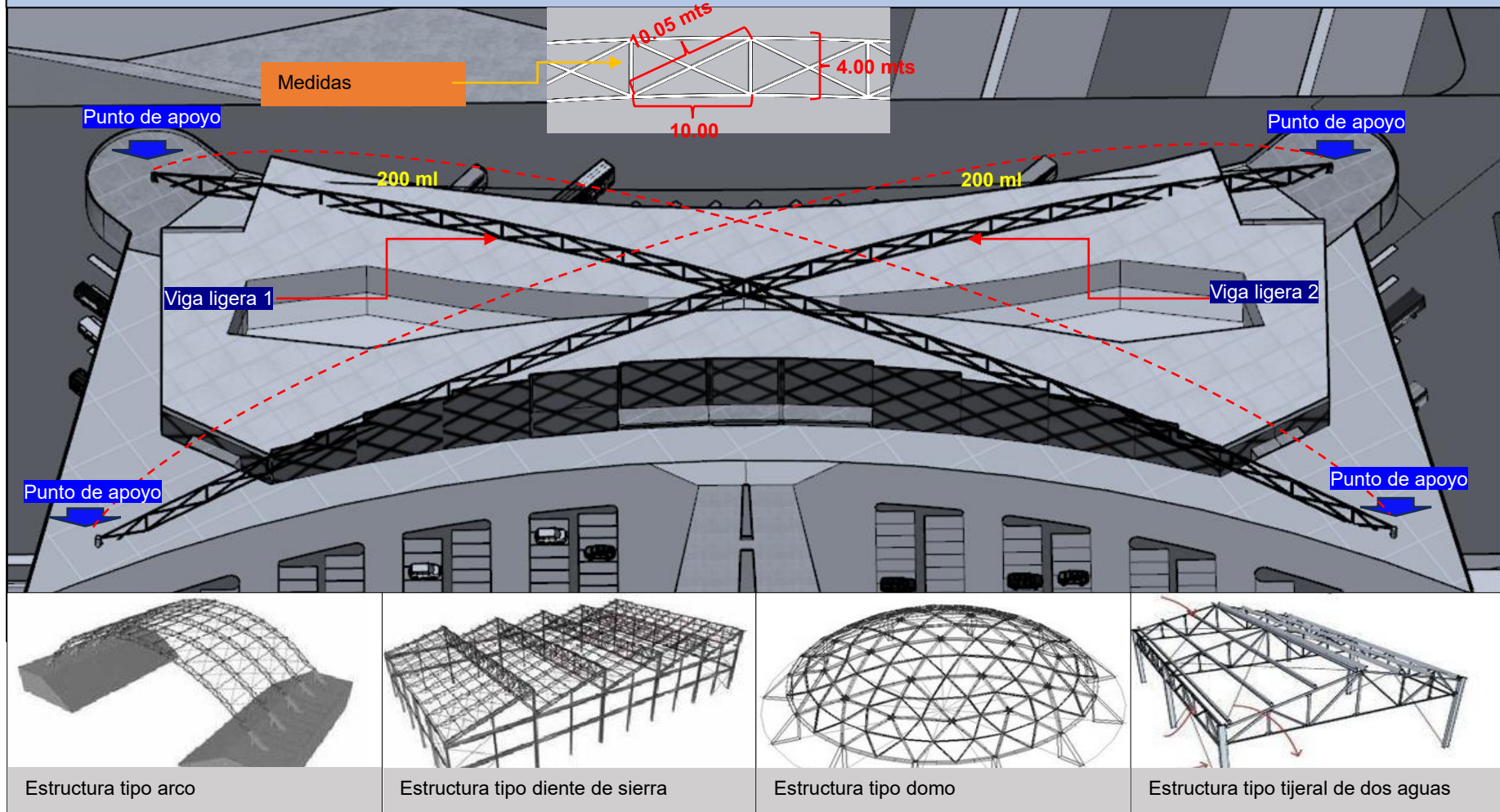
Figura 79. Diseño de la estructura ligera principal.
