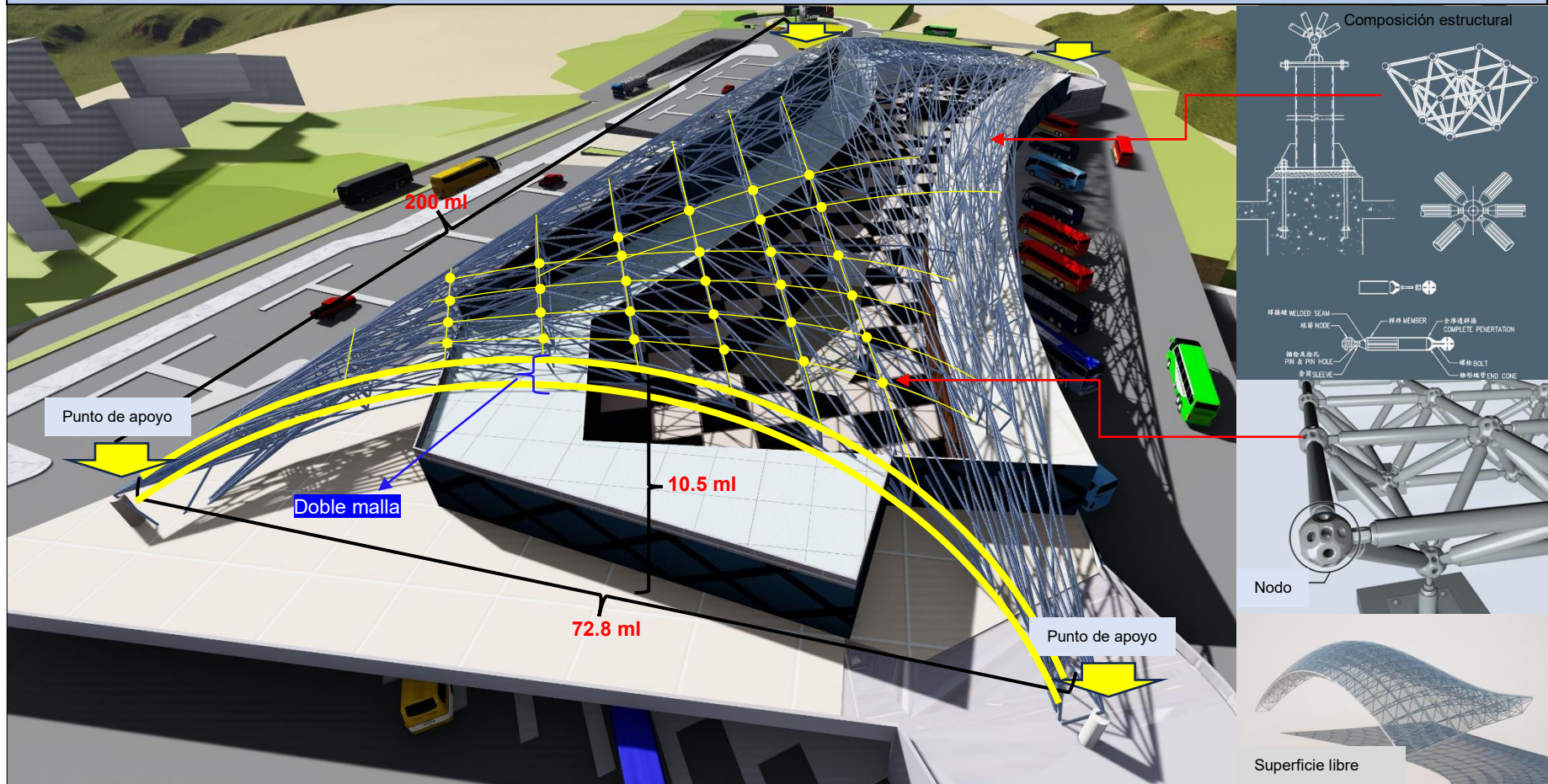
Figura 81. Detalle estructural de la cobertura Diagrid.
