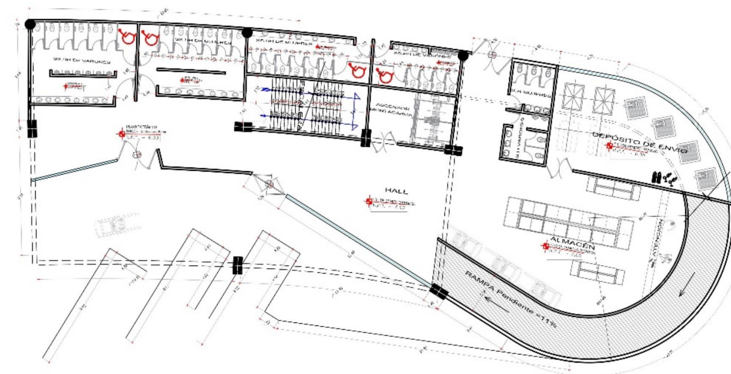
PLANO PRIMER NIVEL - ZONA DE SERVICIOS EMBARQUE ESCALA 1/50
