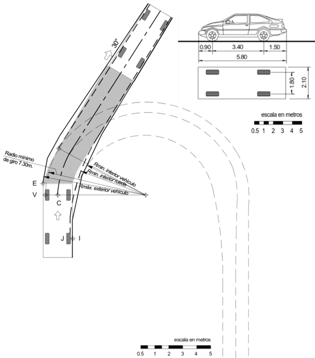
Figura 46. Radios de giro de vehículos ligeros (Fuente: Manual de carreteras Diseño Geométrico DG - 2018).
