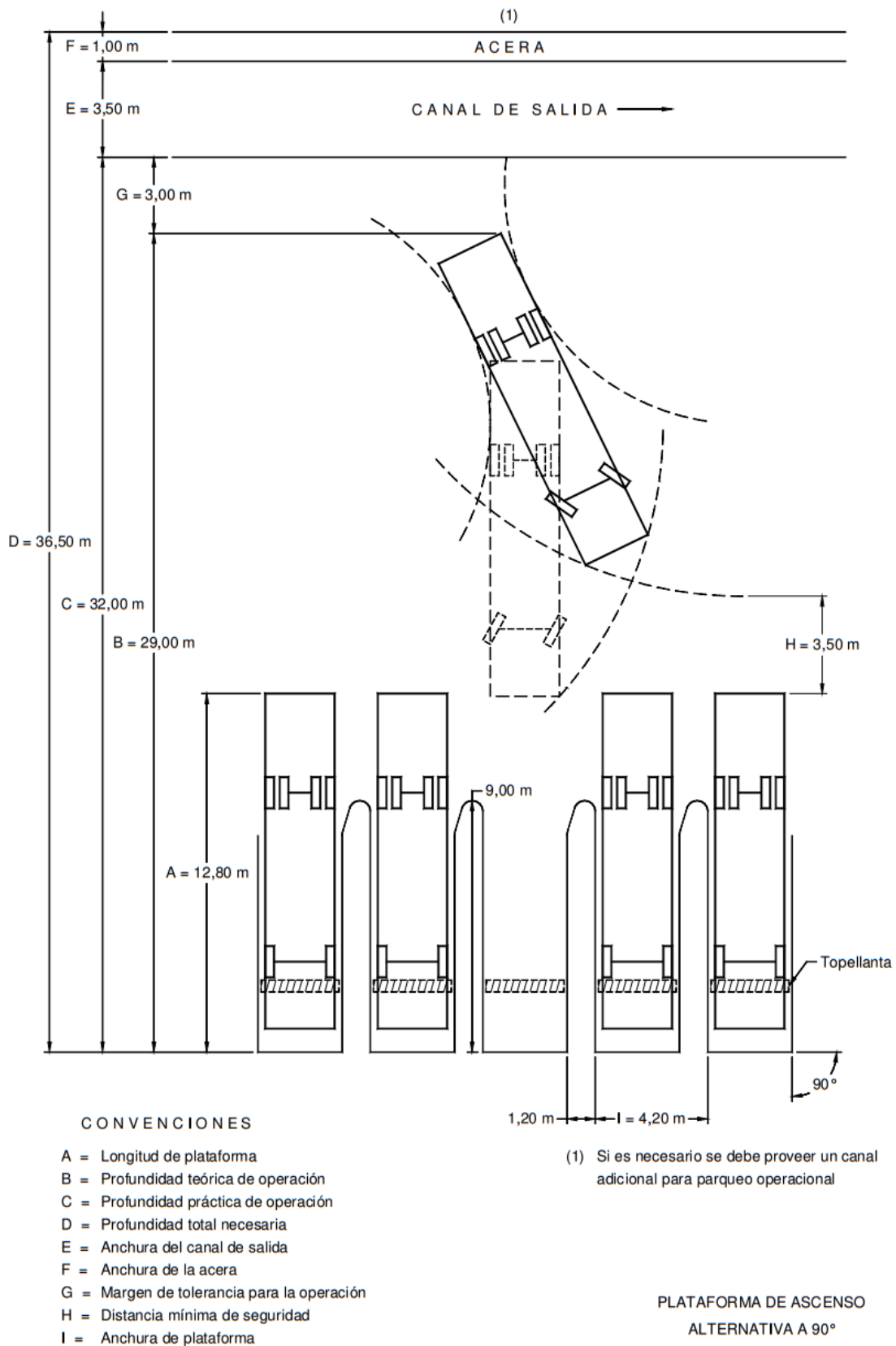
Figura 43. Tipología de medidas y giros en andenes con una inclinación de 90°; (Fuente: Regconomica_Proyecto Norma Técnica Colombiana 430 04).
