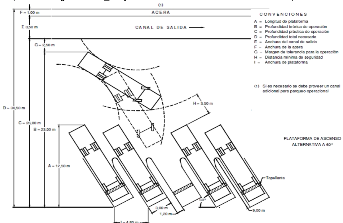
Figura 42. Tipología de medidas y giros en andenes con una inclinación de 60°; (Fuente: Regconomica_Proyecto Norma Técnica Colombiana 430 04).
