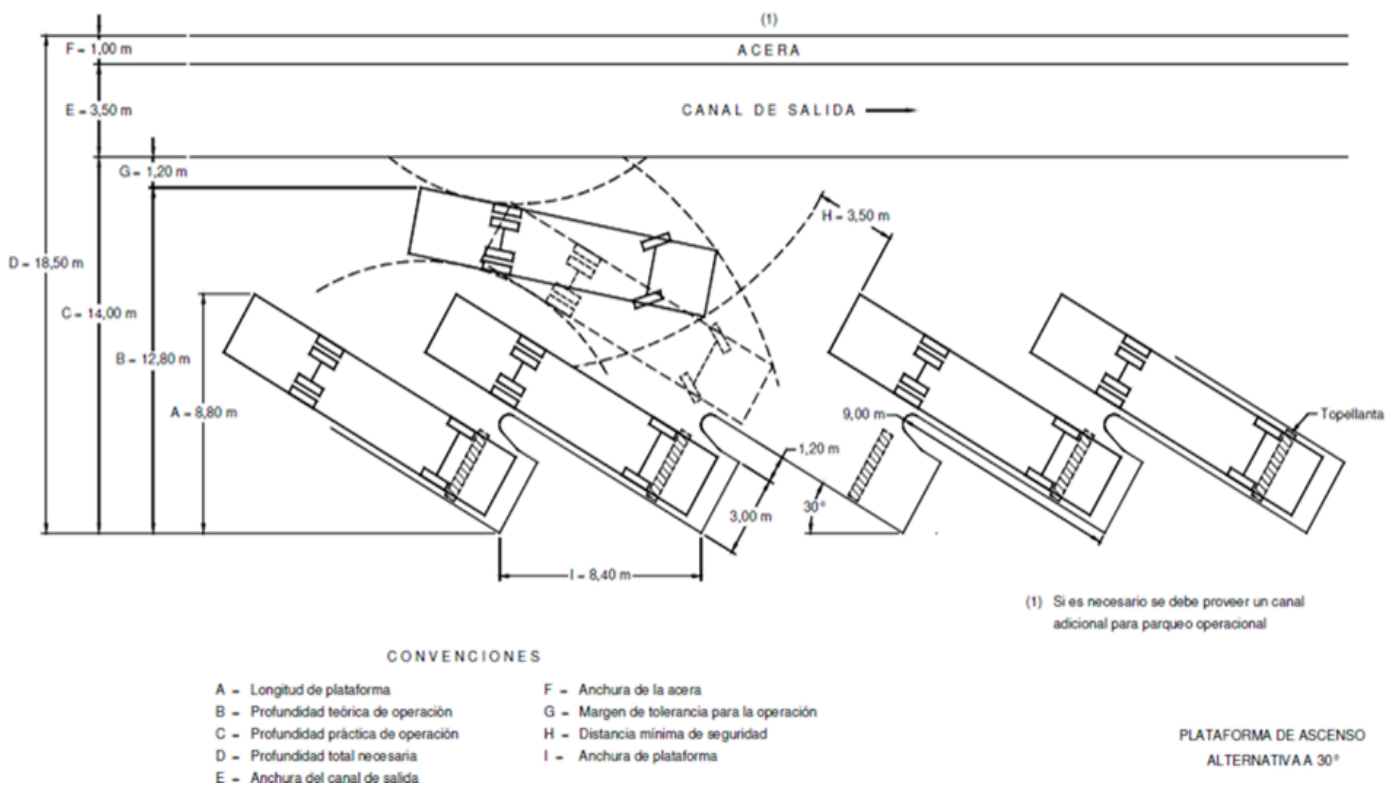
Figura 40. Tipología de medidas y giros en andenes con una inclinación de 30°; (Fuente: Regconomica_Proyecto Norma Técnica Colombiana 430 04).
