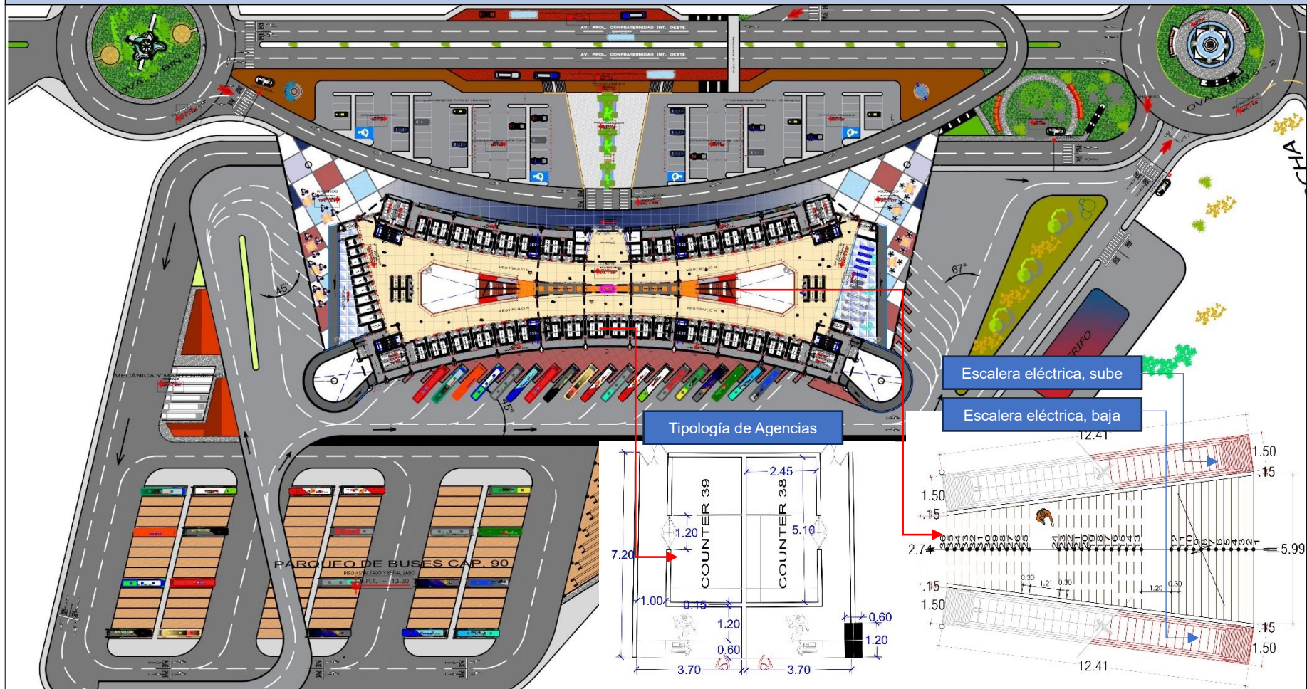
Figura 88. Proceso de diseño; segundo nivel.
