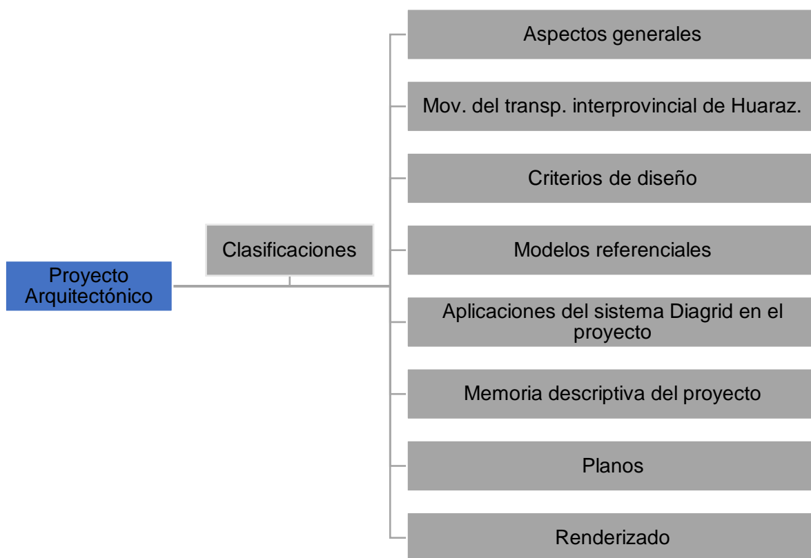
Figura 33. Estructura teórica del proyecto arquitectónico.
