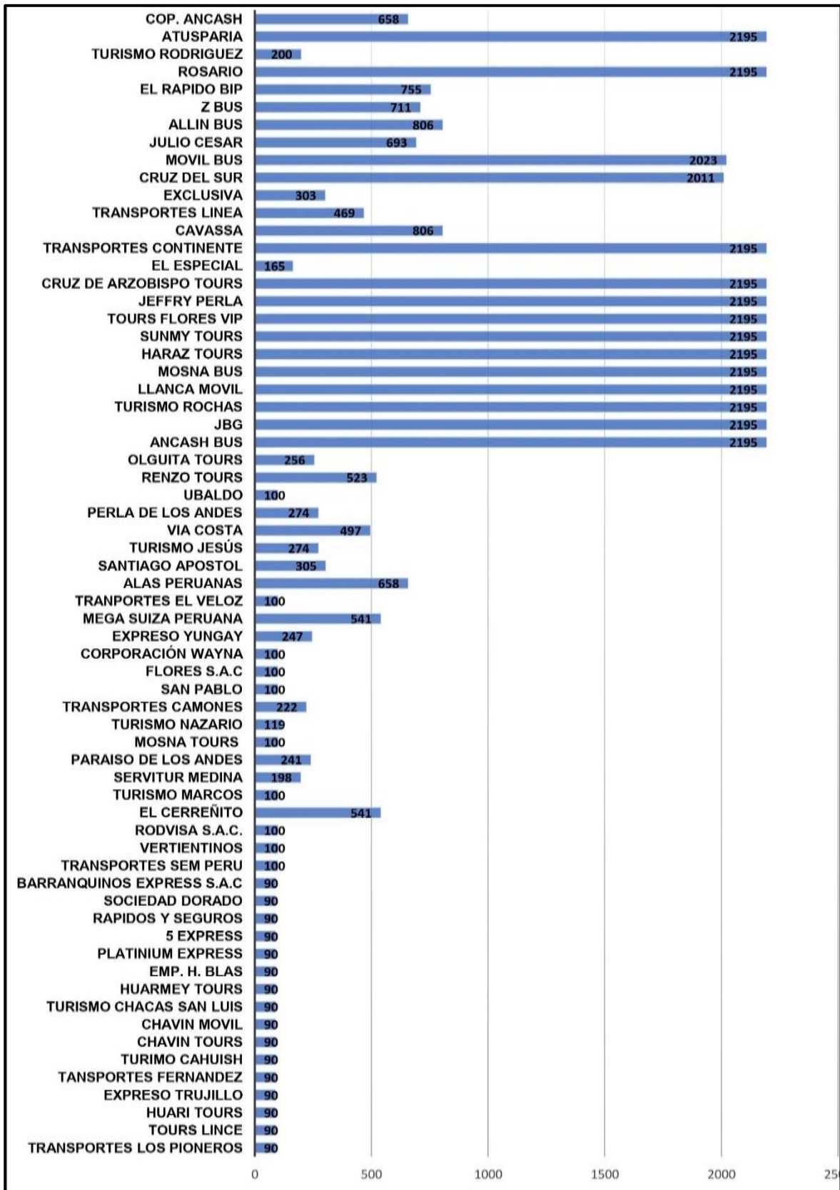
Figura 4. Análisis comparativo general de áreas de las agencias del transporte interprovincial.
