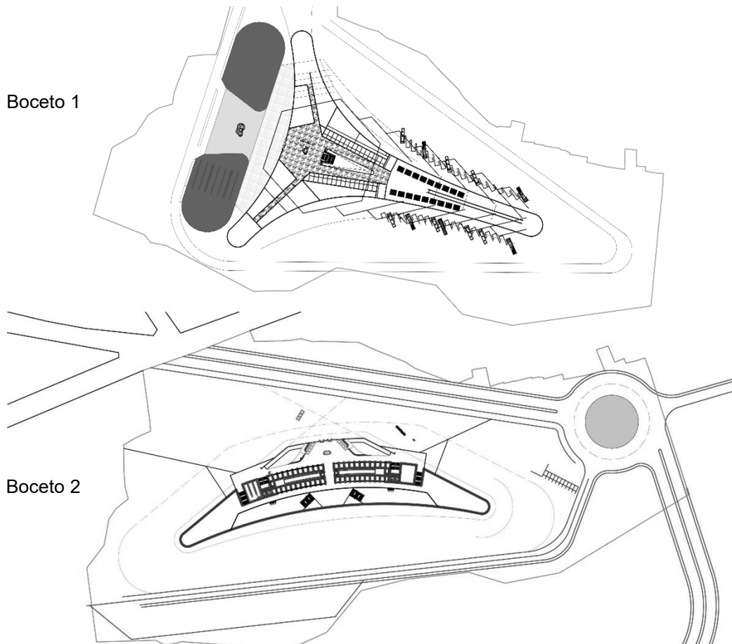
Figura 58. Gráficos del proceso de diseño. Fuente: Elaboración propia, (Araujo Amado, 2023)
