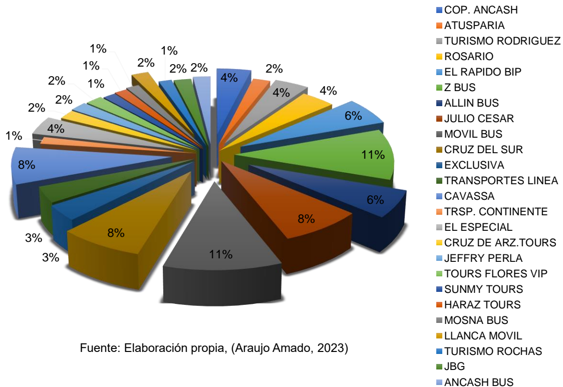
Figura 7. Análisis general; de salidas y llegadas diarias de las empresas del transporte interprovincial en Huaraz.
