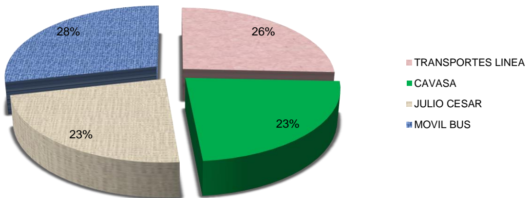
Figura 9. Porcentaje del movimiento de pasajeros por empresa; de acuerdo a salidas diarias referente a la ruta de; Huaraz – Provincias.
