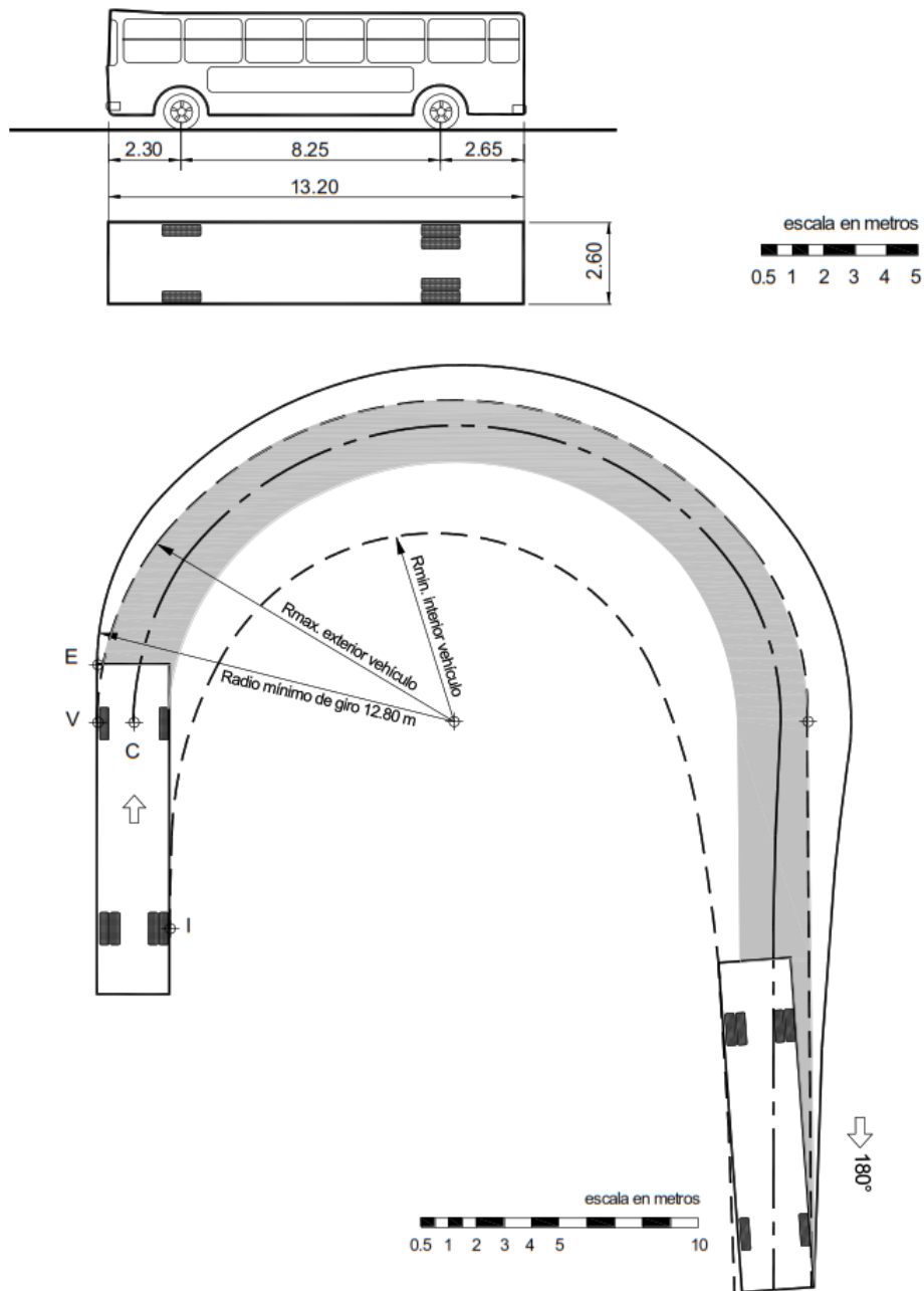
Figura 47. Radios de giro de un Ómnibus de dos ejes (B2); (Fuente: Manual de carreteras Diseño Geométrico DG - 2018).
