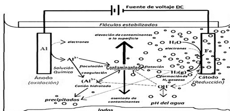
Figura N° 1. Reactor de tipo flujo Fuente: Melgar y Barranco, 2016.
