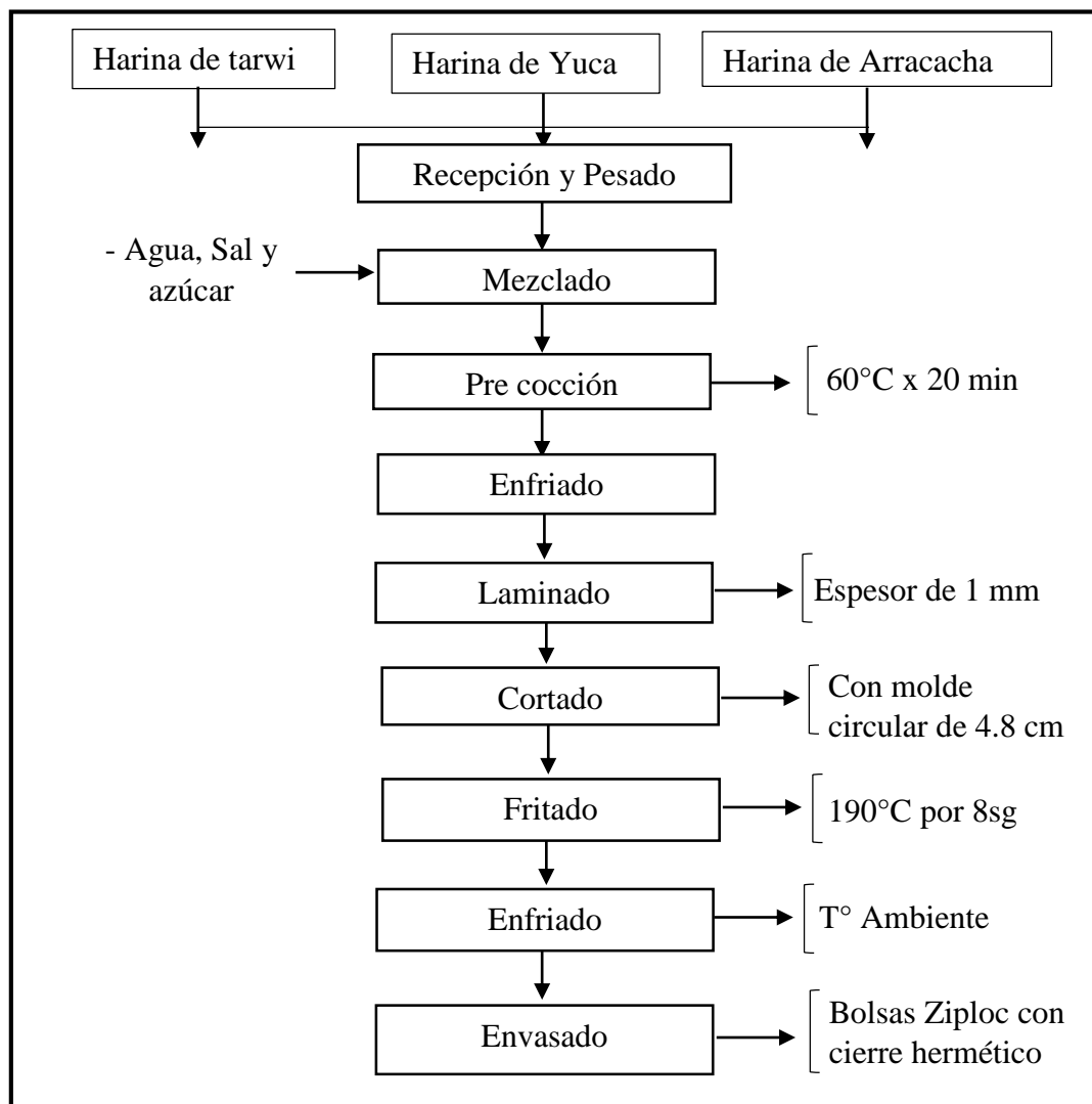
Figura 21: Flujograma para la elaboración de snack a base de harina de tarwi, yuca y arracacha.
