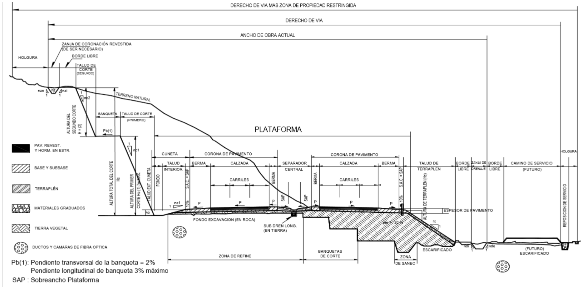
Figura 2: Sección transversal tipo a media ladera para una autopista en tangente
