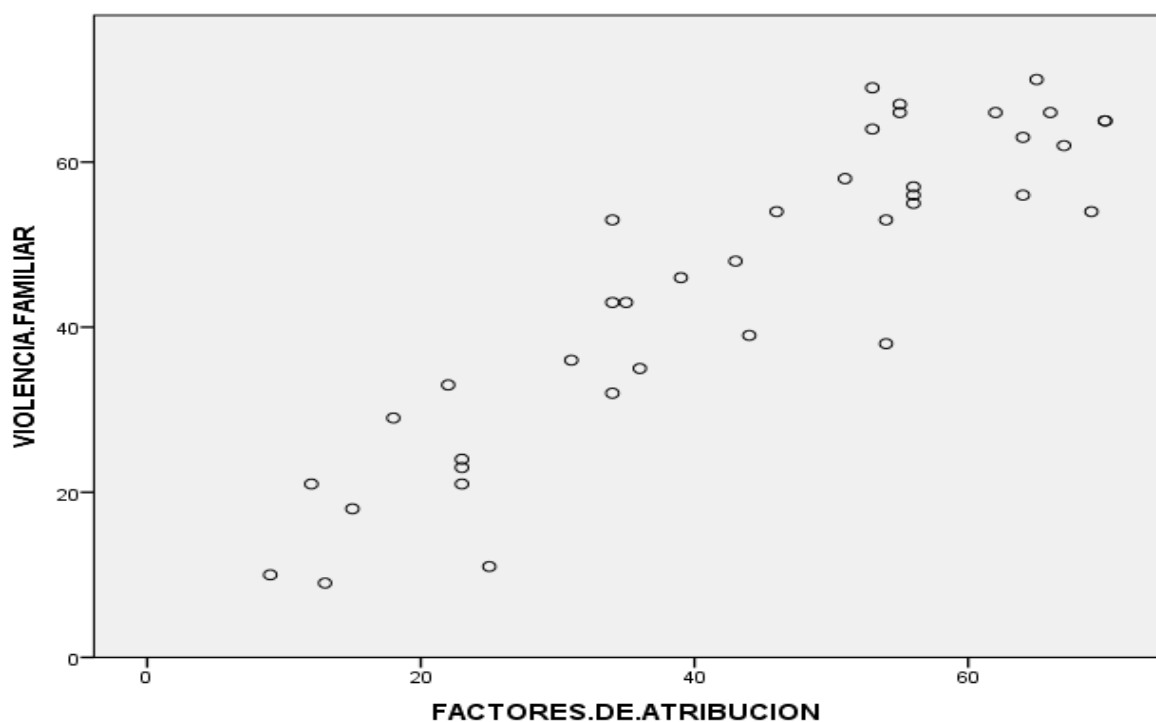
Gráfico 4 de dispersión del problema específico 3
