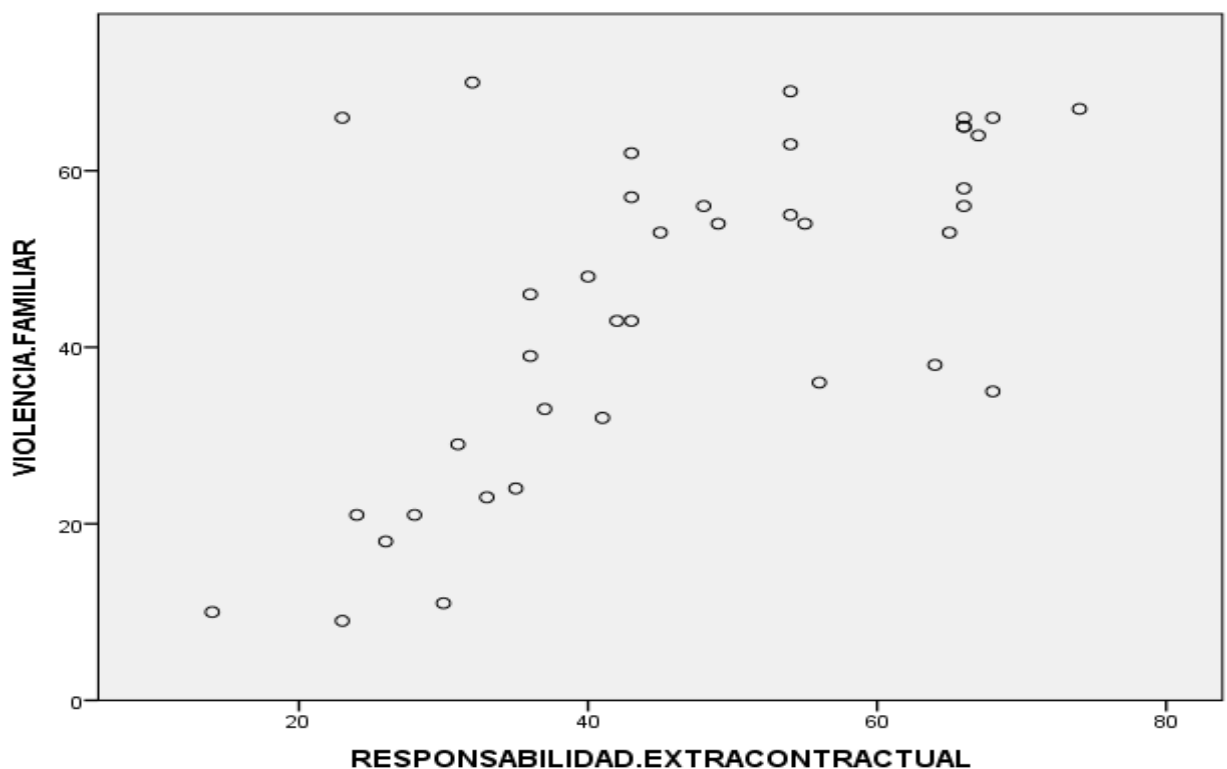
Gráfico 1 de dispersión del problema general
