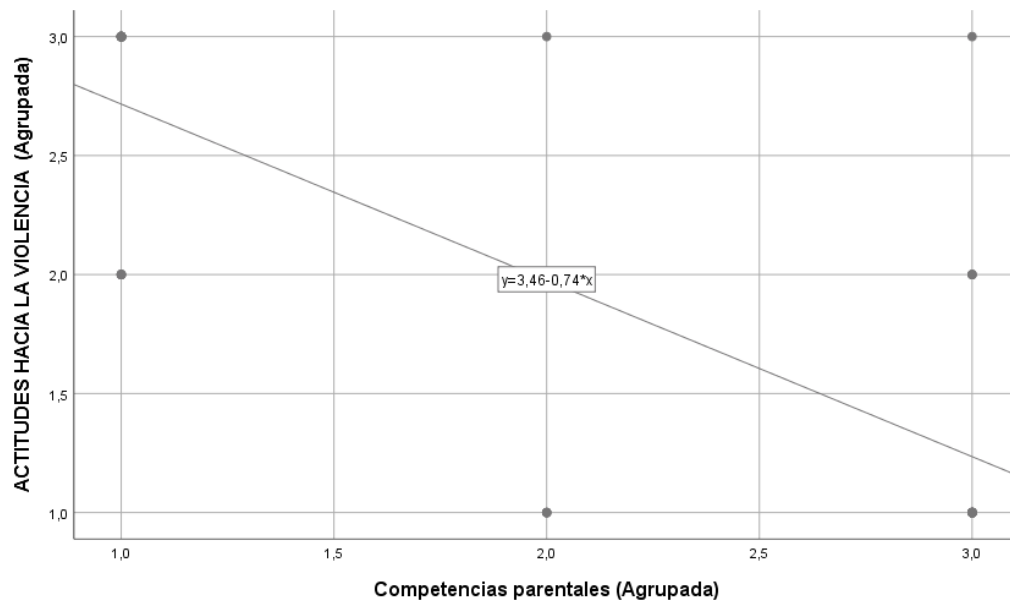
Figura 1 Gráficas de dispersión, actitudes hacia la violencia y competencias parentales
