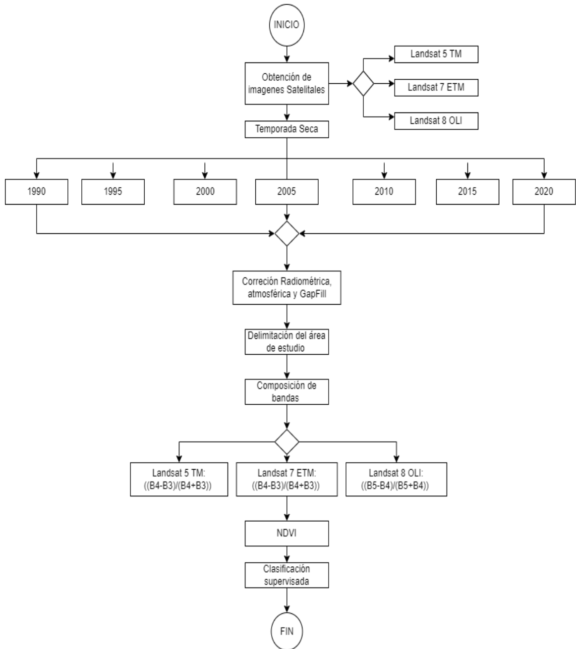
Figura 3. Diagrama de recolección y procesamiento de imágenes satelitales
