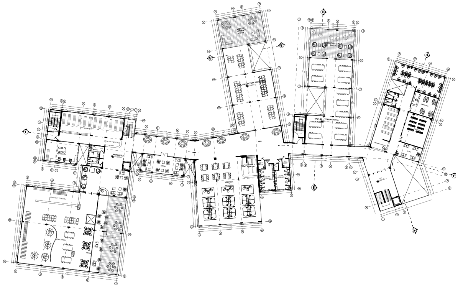
CUARTA PLANTA ESCUELA DE ARTES ESC 1:125
