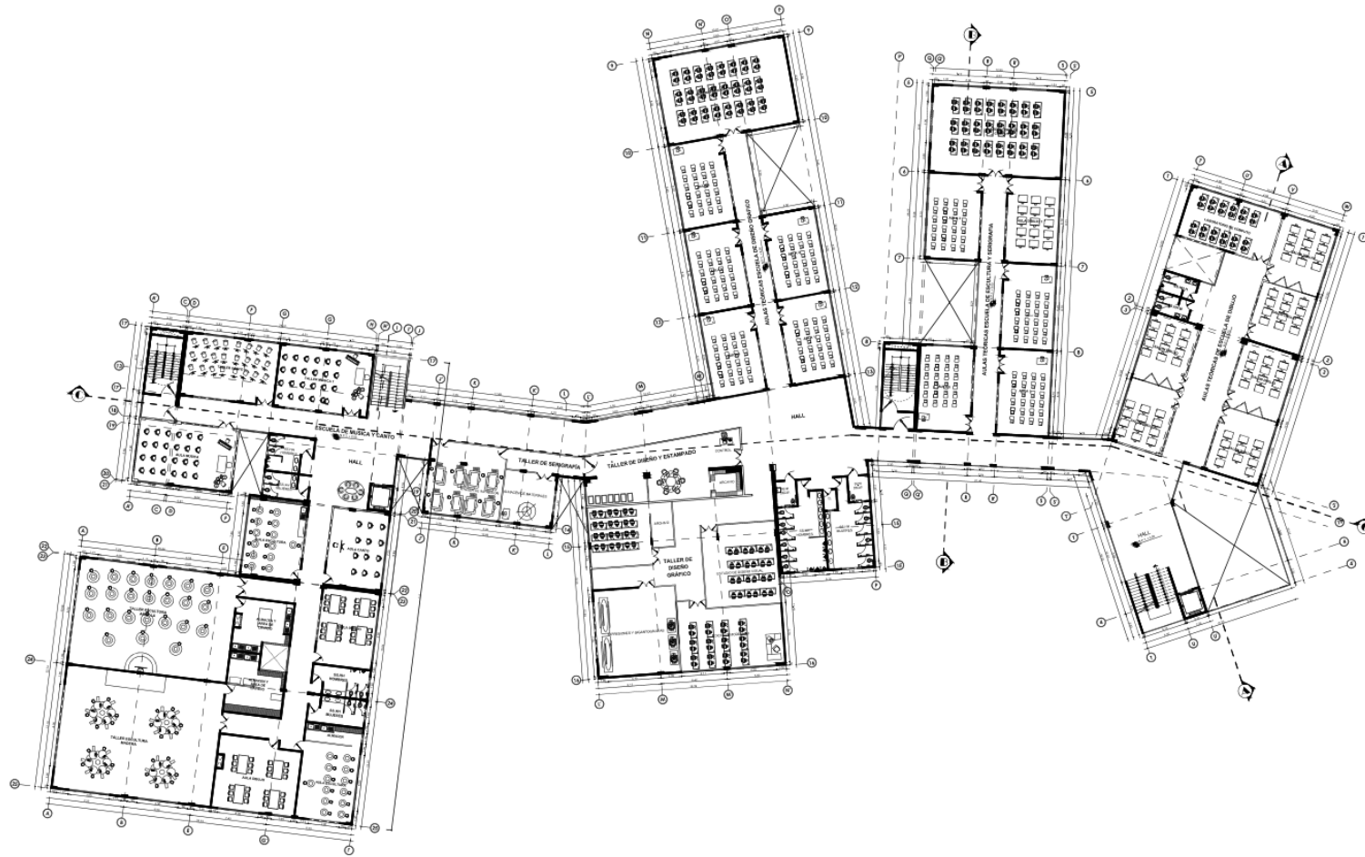
TERCERA PLANTA ESCUELA DE ARTES ESC 1-125
