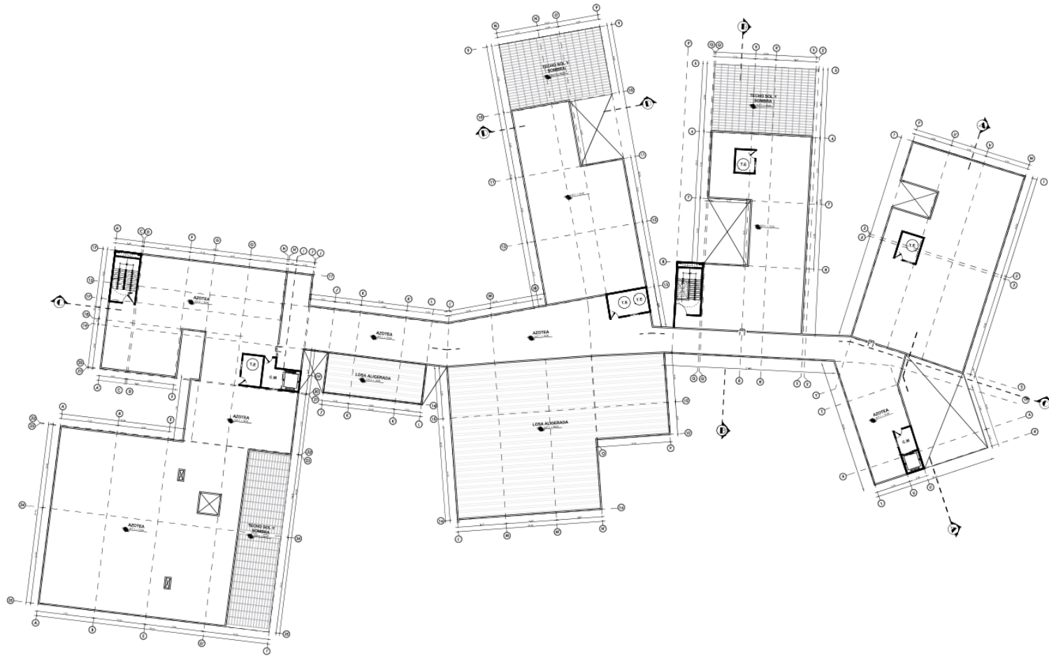
PLANO AZOTEA DE ESCUELA DE ARTES ESC 1:125
