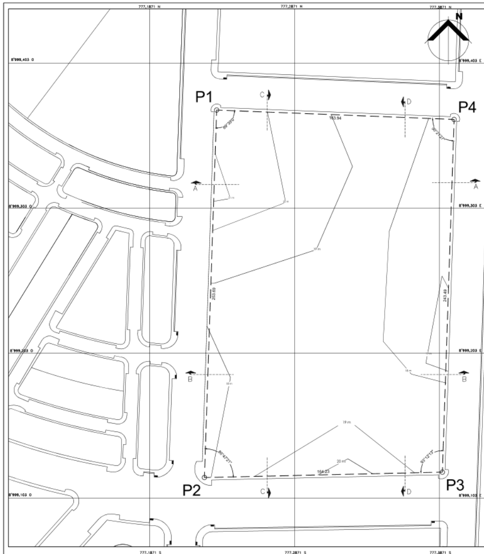
PLANO DE TOPOGRÁFICO ESC: 1/500
