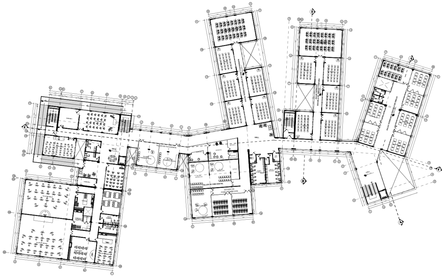
SEGUNDA PLANTA ESCUELA DE ARTES ESQ 1:125
