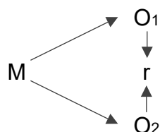
Figura 3: Diagrama del diseño correlacional – causal
