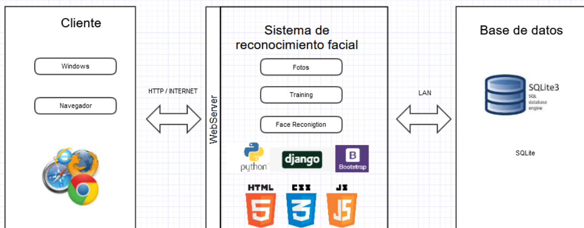
Figura 4 Aquitectura del tecnologica
