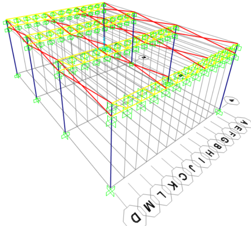
Figura 4 Modelamiento 3D estructura metálica
