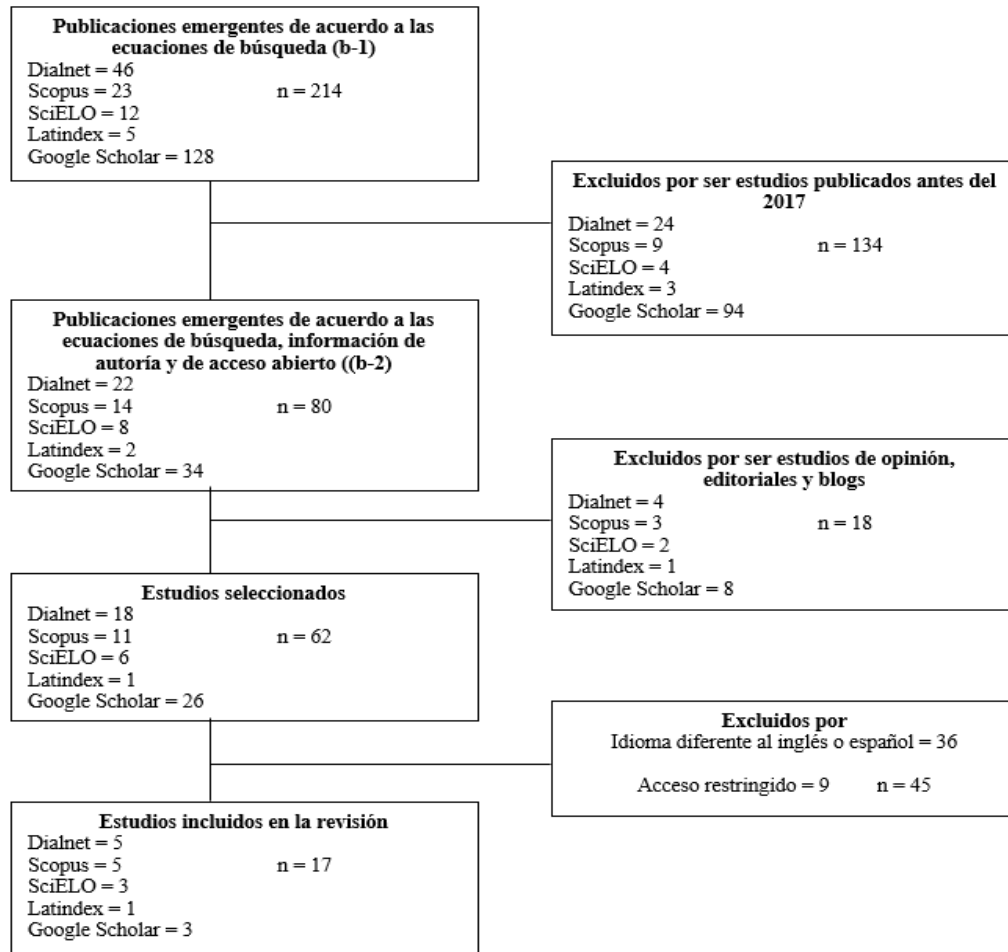
Figura 1. Flujograma PRISMA
