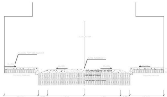
SECCION DE LA CALLE 1,2,3,4 ESC. 1/50
