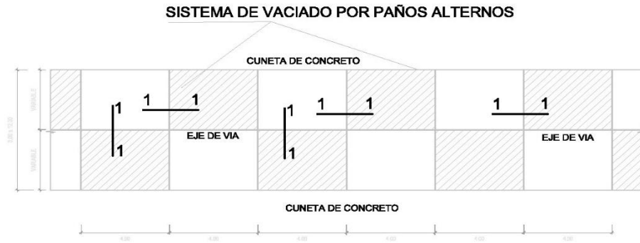
DISTRIB. DE PAÑOS ESC. 1/100
