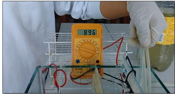
Figura A4: Medición de MiliVoltios en la celda microbiana agregando 1,398 (L/min) de oxígeno.
