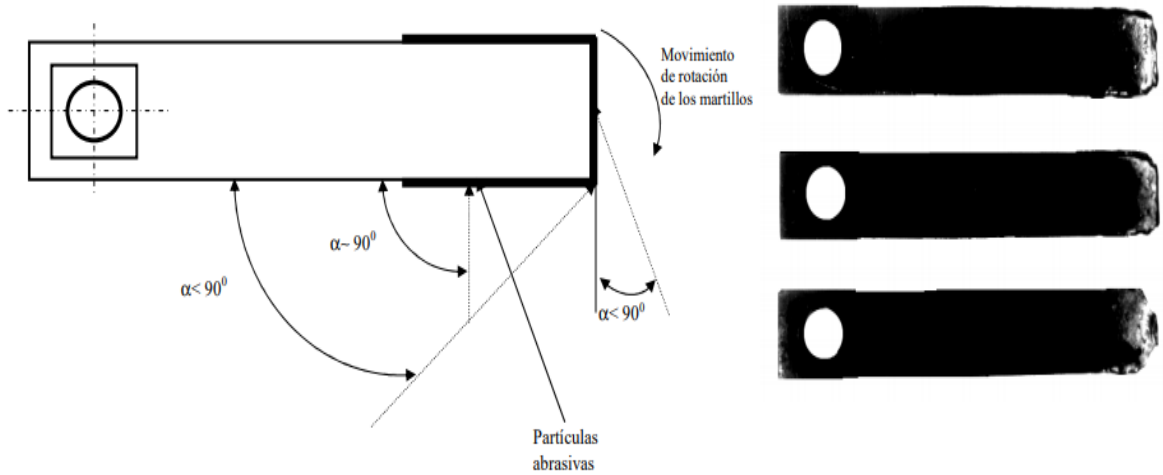
FIGURA Nº 8: Cuchillas de Molinos Recubrimiento con UTP-711 (Carburos de Cromo Formando Redes) (J. Gómez 2004)
