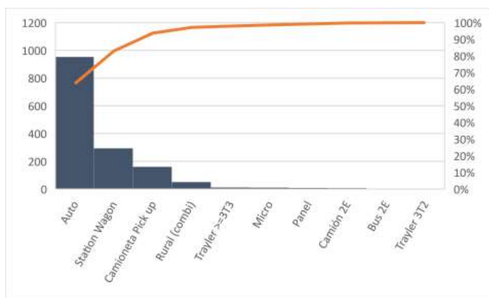
Gráfico N° 04. IMDA (Veh/día)
