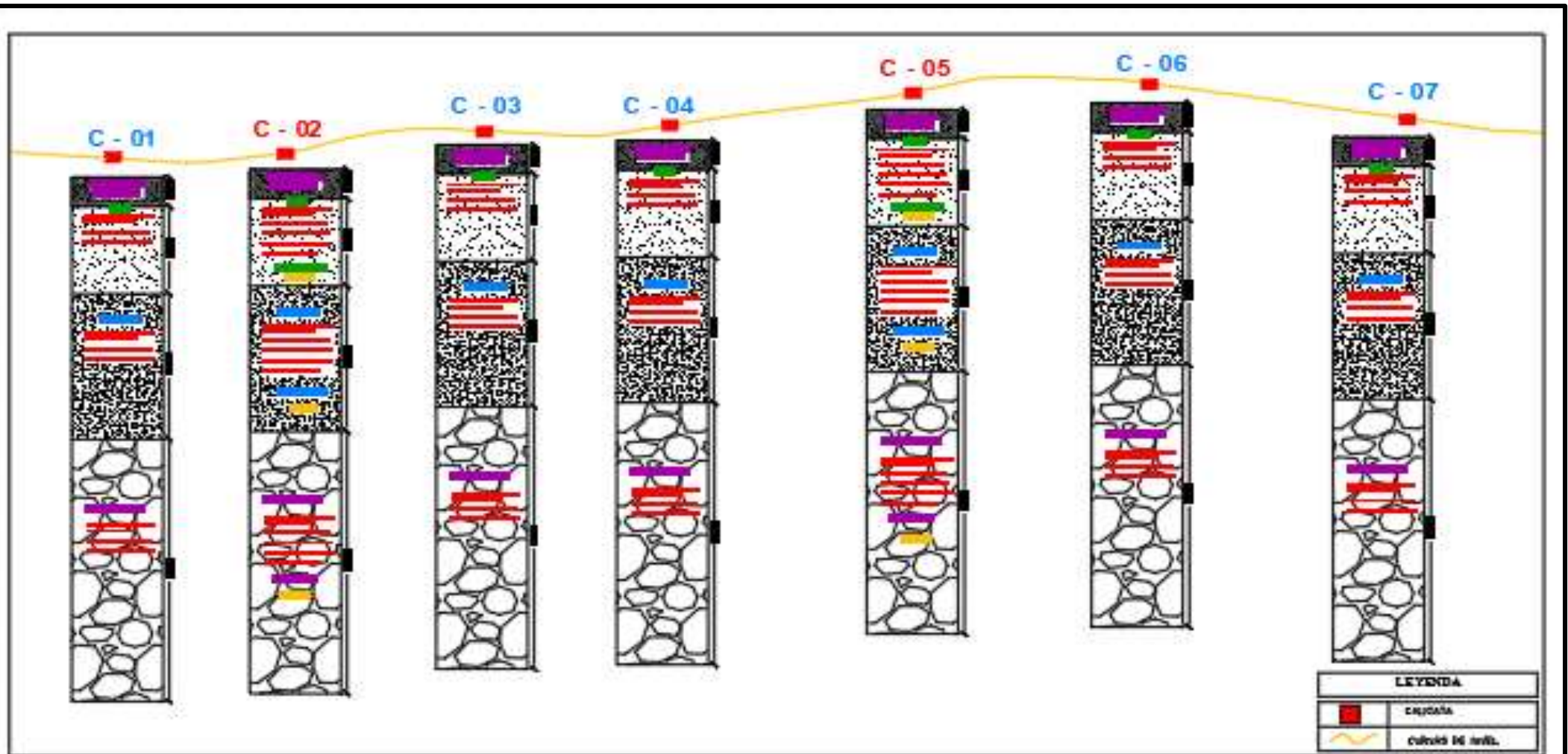
PERFIL ESTATIGRÁFICO ESCALA 1/10
