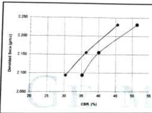
EC = 86 GOLPES
