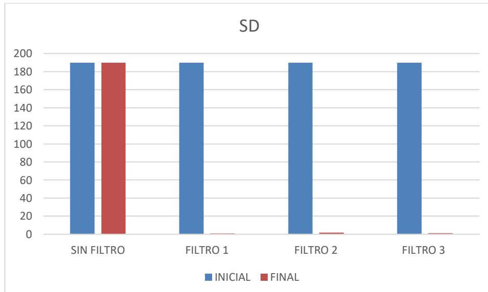
Gráfico 3 Resultados de Sólidos Disueltos
