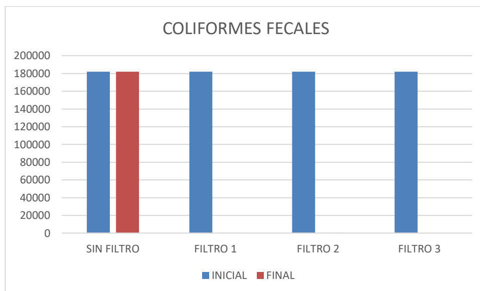
Grafico 12 Resultados de coliformes
