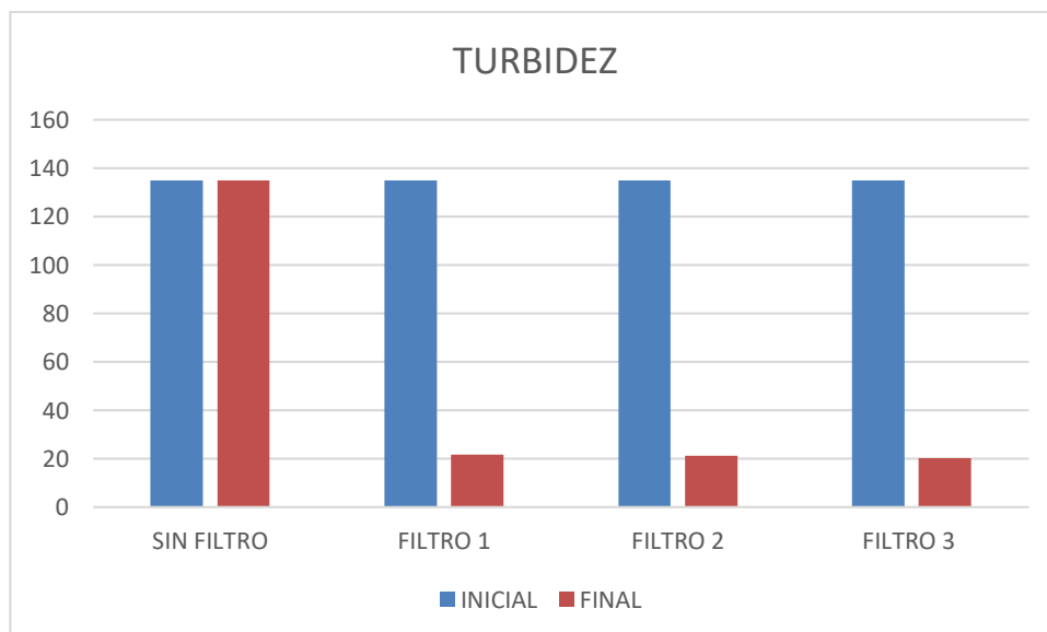
Grafico 5 Resultados de Turbidez
