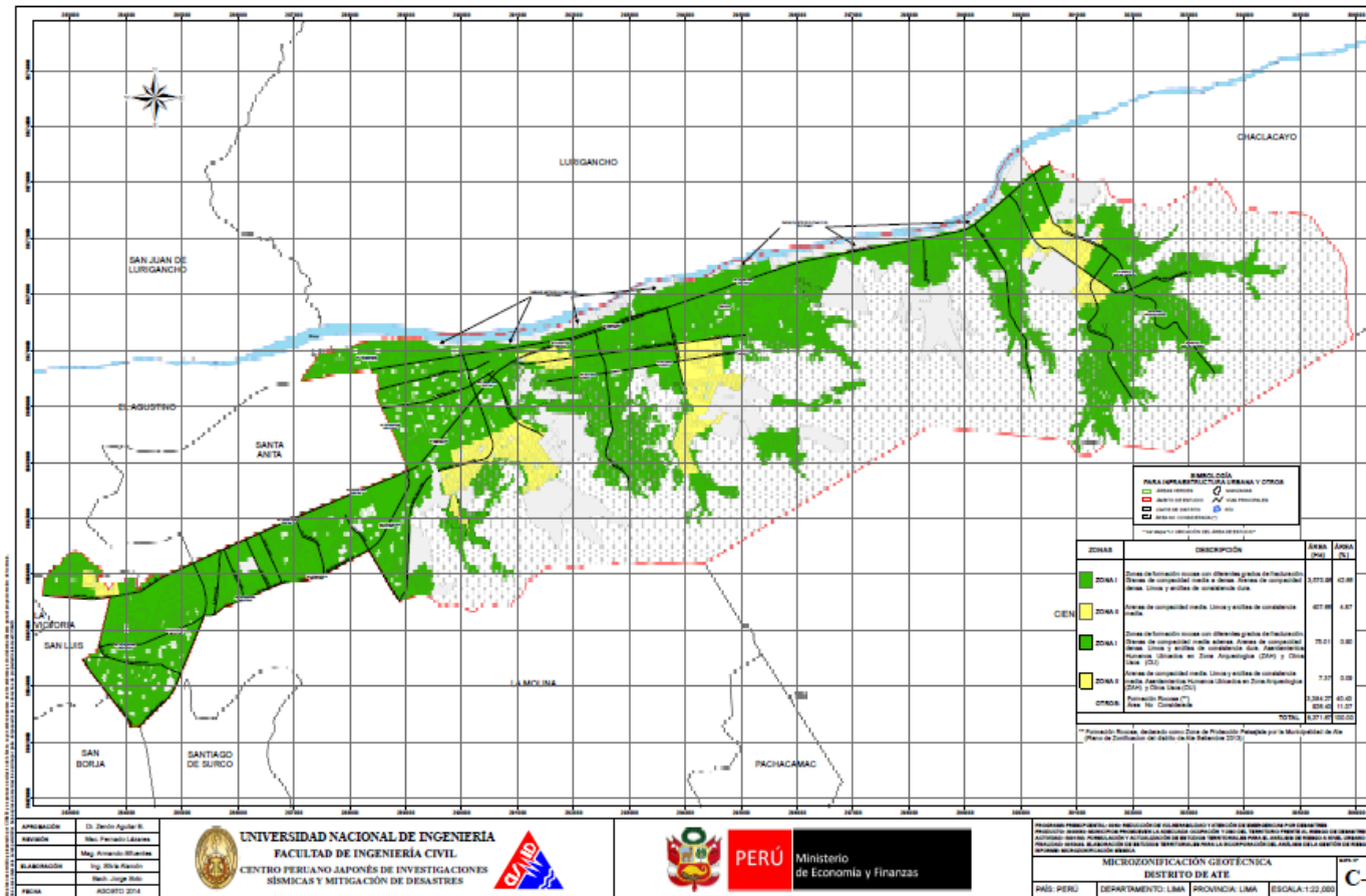
Fig. 16 Mapa de microzonificación geotécnica distrito de Ate – Cismid
