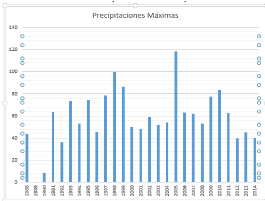
Figura 3. Precipitaciones máximas por año
