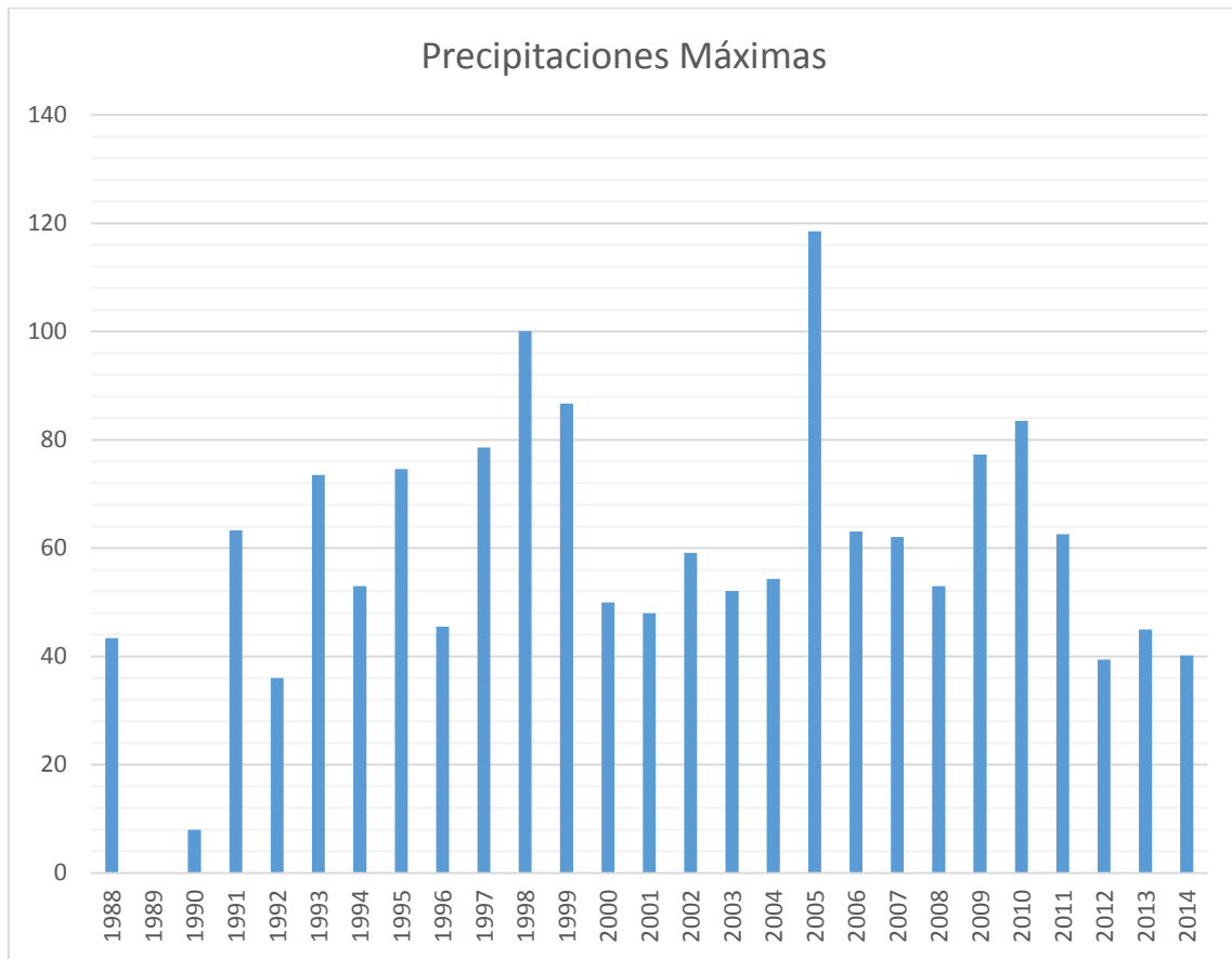
Gráfico 1. Precipitaciones máximas por año.
