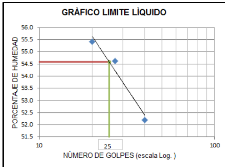
Figura 23. Esquema para decretar el Límite Líquido
